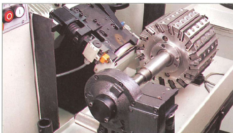
▲ Ein Hydro-Rotaplan-Messerkopf mit Schneiden wird rundgeschliffen. Höchste Genauigkeit: Schleifen eines Hydro-Fräsers. ▶
