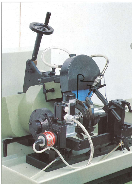
▲ Ein Hydro-Rotaplan-Messerkopf mit Schneiden wird rundgeschliffen. Höchste Genauigkeit: Schleifen eines Hydro-Fräsers. ▶
