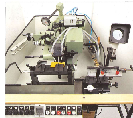
Profilschablone fertigen.
