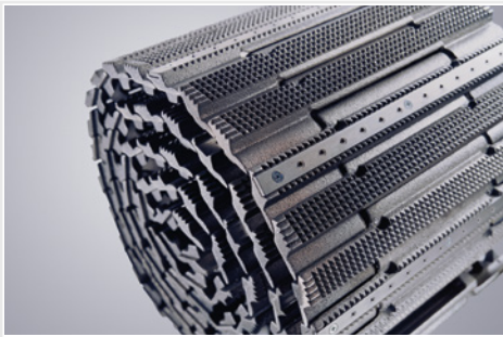
Geschlossene Vorschubkette – zuverlässiger Holztransport
