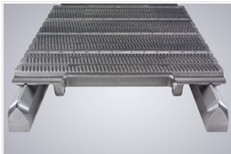
Prismengeführte Vorschubkette: beste Schnittergebnisse
