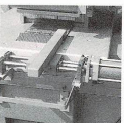
Pneumatikverstellung Einlauflineal 2 Positionen pneumatic guiding fence adjustment for 2 positions
